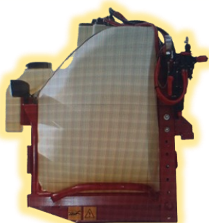
Cuve Physeter 750 litres
